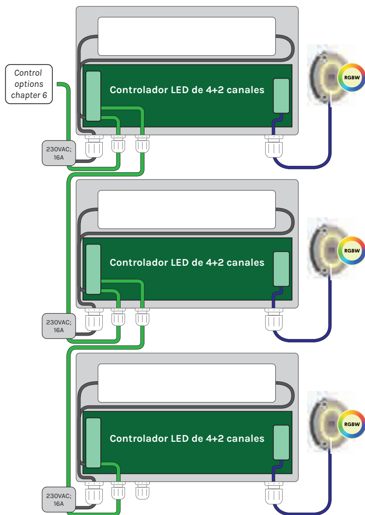
Vista general - Combinación de lámparas subacuáticas LED RGBW y fuentes de alimentación
